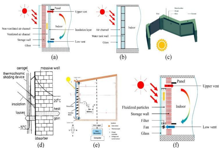
شکل ۲: پیکربندی‌های مختلف دیوار ترومب: (الف) TW کامپوزیت [۱۹]، (ب) TW آب [۲۰]، (ج) TW زیگزاگ، (د) TW ترموکرومیک [۲۱]، TW فتوولتائیک [۲۲] و TW (ع) سیال شده [۱۹].
