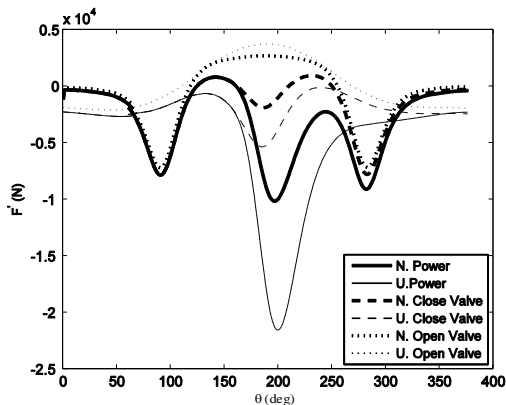
شکل ۱۴) نمودار نیروهای وارده بر شاتون-زاویه لنگ، در شرایط احتراق و بدون احتراق با سوپاپ بسته و باز در مکانیزمهای مرسوم و
