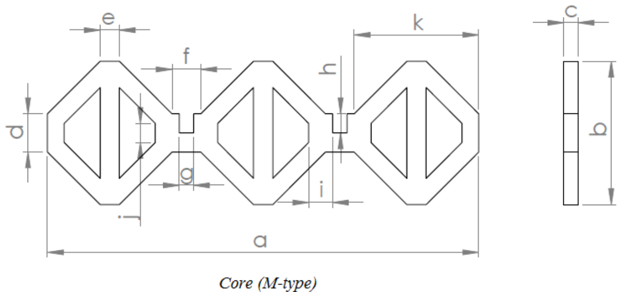
شکل ۳: ابعاد و اندازه های هسته‌ی ساندویچ پانل
