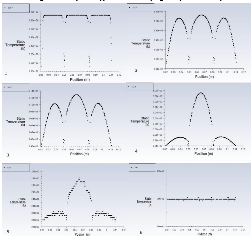
شکل ۱۴: تغییرات دما در طول خط در گذر زمان
