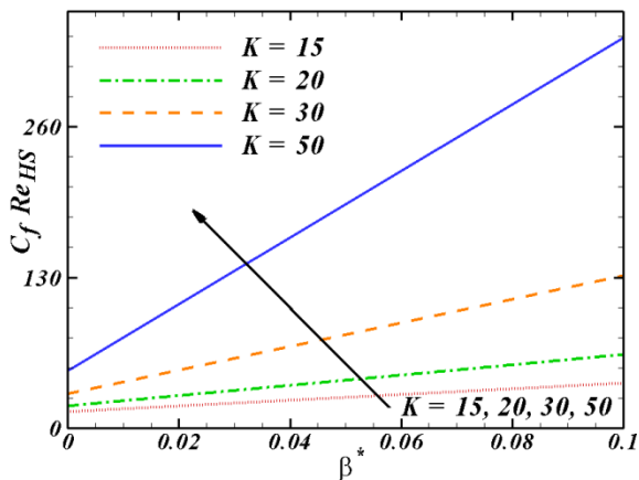
شکل ۳۷: تأثیر پارامتر دمای K بر C_f Re_{HS} ، به ازای A = 1 و 1
