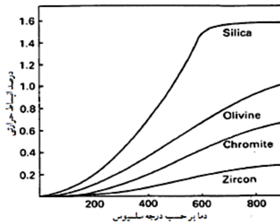
شکل ۴: نمودار مقایسه‌ای میزان ضریب انبساط حرارتی ماسه‌های الیومینی با ماسه‌های سیلیسی، کرومیتی و زیرکونیایی [۱۱]
