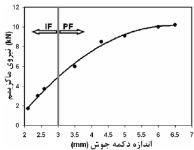
شکل (۳): تغییرات نیروی ماکزیمم و مود شکست بر حسب اندازه دکهه جوش [۵]
