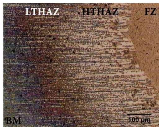
شکل (۸): ریز ساختار منطقه‌ی متأثر از حرارت (HAZ) فولاد دوبلکس
