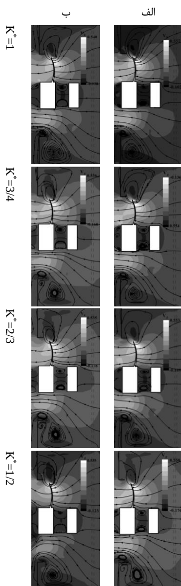
ادامه شکل ۱۲: سرعت بی‌بعد محوری و خطوط جریان عبوری از واحد بیرونی و میانه فن جریان محوری با ضریب نفوذپذیری مختلف (الف) ۸۲۰ دور بر دقیقه (ب) ۵۲۰ دور بر دقیقه
