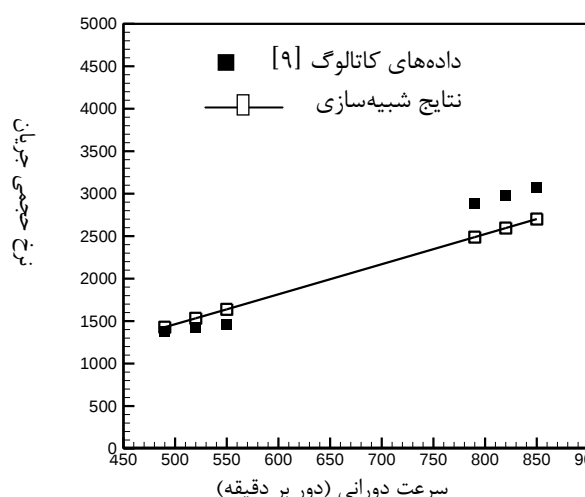
شکل ۷: تغییرات نرخ حجمی جریان بر حسب سرعت دورانی
