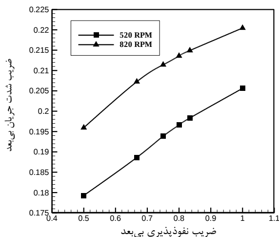
شکل ۱۴: تغییرات ضریب شدت جریان بی بعد بر حسب ضریب نفوذ پذیری بی بعد
