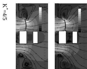
شکل ۱۲: سرعت بی‌بعد محوری و خطوط جریان عبوری از واحد بیرونی و میانه فن جریان محوری با ضریب نفوذپذیری مختلف (الف) ۸۲۰ دور بر دقیقه (ب) ۵۲۰ دور بر دقیقه
