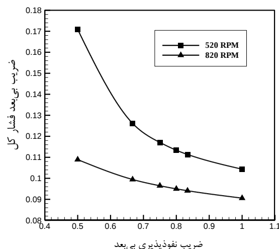
شکل ۱۳: تغییرات ضریب بی بعد فشار کل بر حسب ضریب نفوذ پذیری بی بعد
