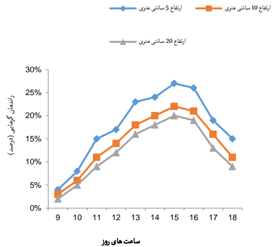
شکل ۱۱: نمودار مقایسه تغییرات راندامان گرمایی در سه ارتفاع ۵، ۱۰ و ۲۰ سانتی متری در ساعات های مختلف روز بدون جریان اجباری
