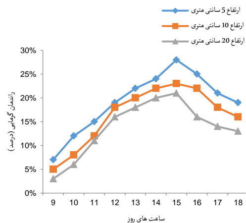
شکل ۱۲: نمودار مقایسه تغییرات راندمان گرمایی در سه ارتفاع ۵، ۱۰ و ۲۰ سانتی متری در ساعات های مختلف روز با جریان اجباری
