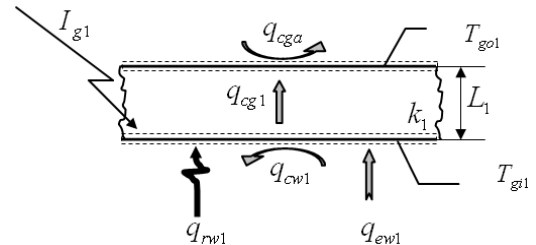
شکل ۳: نمای شماتیک پایداری انرژی در پوشش شیشه ای [22]
