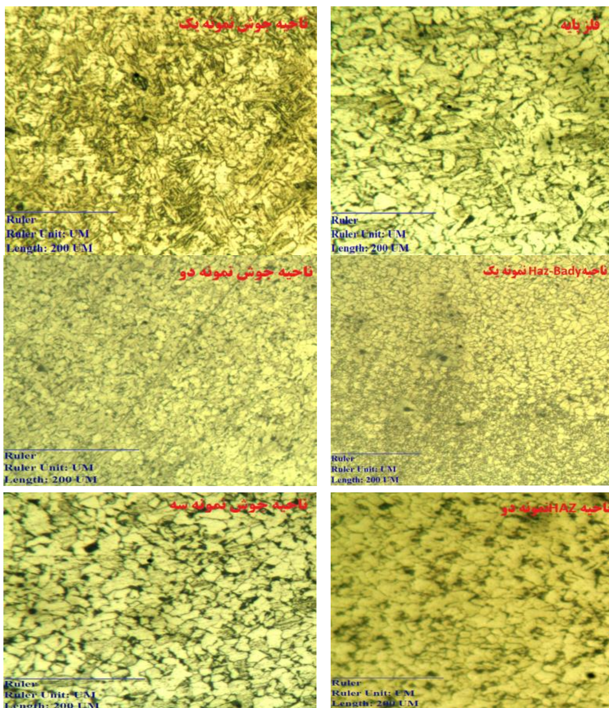
شکل ۳: تصاویر متالوگرافی از فلز پایه و نمونه‌های ۱، ۲ و ۳
