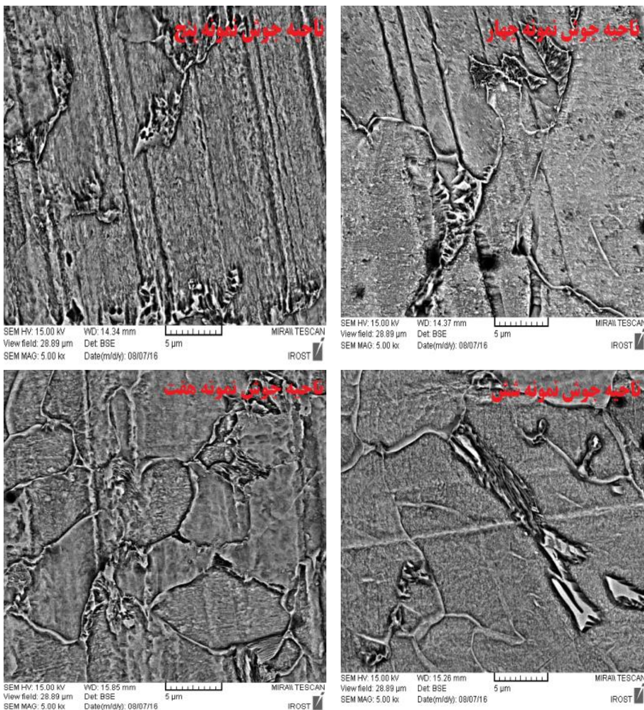
شکل ۶: تصاویر SEM نمونه‌های ۴، ۵، ۶ و ۷
