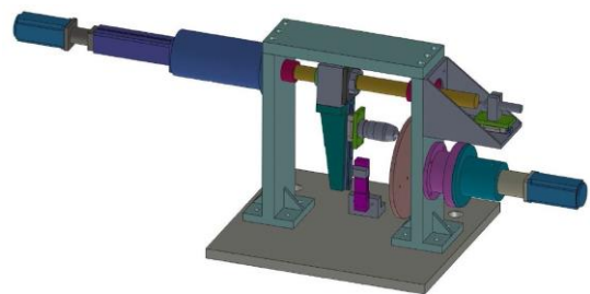
شکل ۱: دستگاه تست سایش به صورت شماتیک
