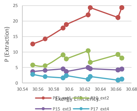
شکل ۹: تاثیر تغییرات فشارهای زیرکش توربین بر بازده اگزرژی
