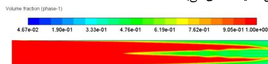
شکل (۴) کسر حجمی مایع در صفحه میانی ( q=7500 \text{ w/m}^2 )
