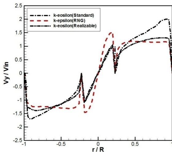
شکل ۶: مقایسه سرعت y در مقطع ۳ برای سه مدل آشفتگی
