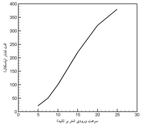
شکل ۷: افت فشار در سیکلون بر حسب سرعت ورودی [۱۰]
