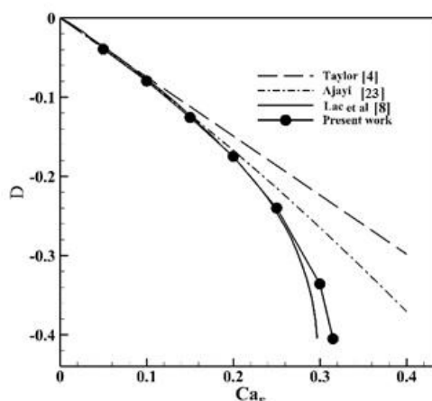
شکل ۸- تغییر شکل آبلیت قطره نیمه‌رسانا در اعداد موینگی الکتریکی مختلف برای \epsilon_r = 2 و \sigma_r = 0.1
