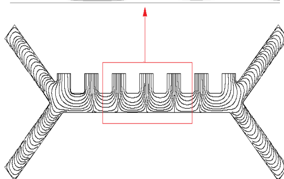
شکل ۷- الف) توزیع پتانسیل الکتریکی و ب) توزیع خطوط میدان الکتریکی.
