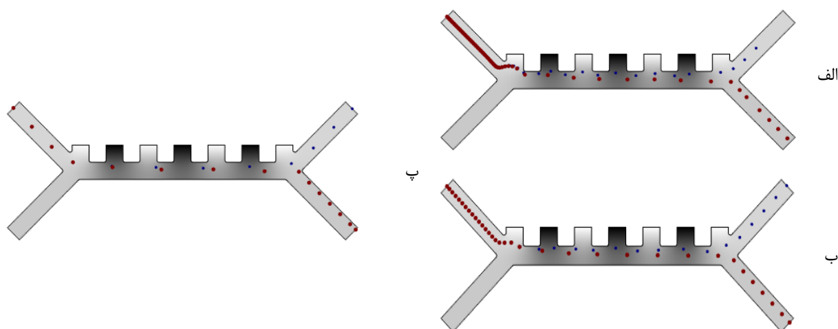
شکل ۸- تغییرات سرعت در ورودی میکروکانال در فرکانس ۱۰۰ KHz، ولتاژ ۵V و سرعت ورودی محلول بافر 900 \mu\text{m/s} در زمان ۳ ثانیه برای سرعت ذرات متفاوت: الف) 70 \mu\text{m/s} ، ب) 150 \mu\text{m/s} و پ) 900 \mu\text{m/s} .
