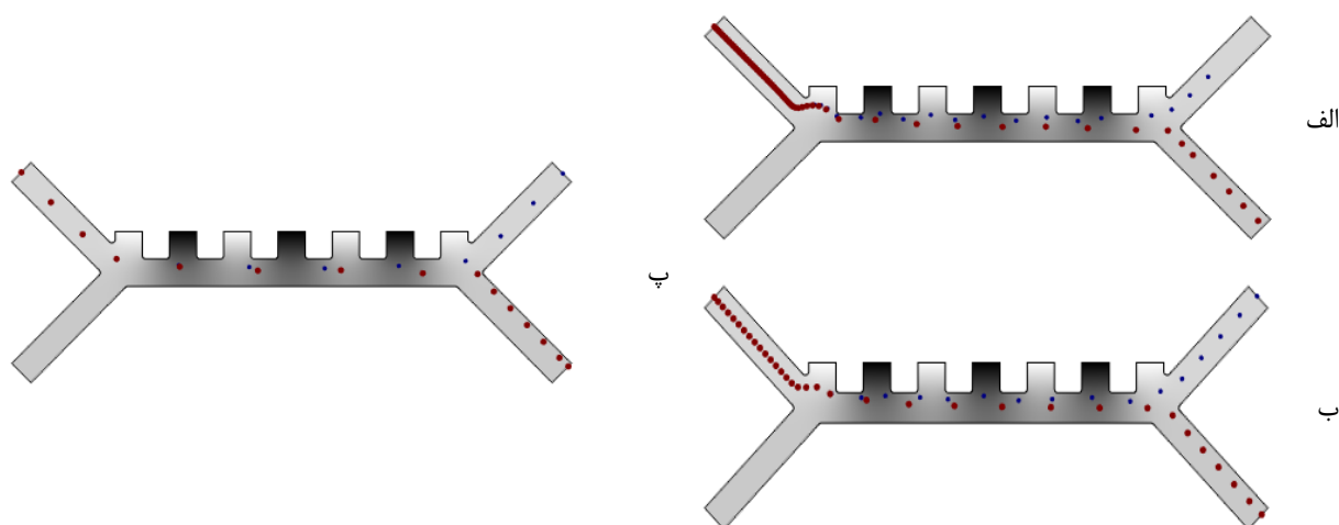
شکل ۸- تغییرات سرعت در ورودی میکروکانال در فرکانس ۱۰۰ KHz، ولتاژ ۵V و سرعت ورودی محلول بافر 900 \mu\text{m/s} در زمان ۳ ثانیه برای سرعت ذرات متفاوت: الف) 700 \mu\text{m/s} ، ب) 1500 \mu\text{m/s} و پ) 900 \mu\text{m/s} .
