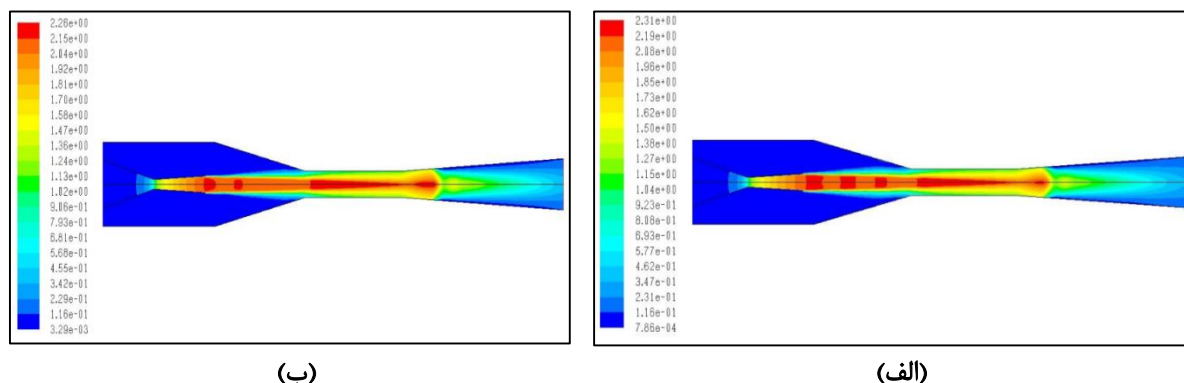
شکل ۱۳- کانتور عدد ماخ برای سیال عامل R۱۴۱b و دمای اواپراتور 12^\circ\text{C} و دمای ژنراتور الف: 78^\circ\text{C} ب: 95^\circ\text{C}
