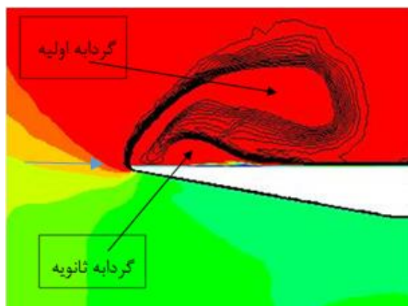
شکل ۶- کانتور ماخ و خطوط فشار ثابت در مقطع ۹۰٪ برای حالت M=1.2 \alpha=30^\circ , \Lambda=65^\circ
