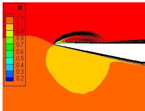
شکل ۵- کانتور ماخ و خطوط فشار ثابت در مقطع ۹۰٪ برای حالت M=1.2 \alpha=8^\circ , \Lambda=65^\circ
