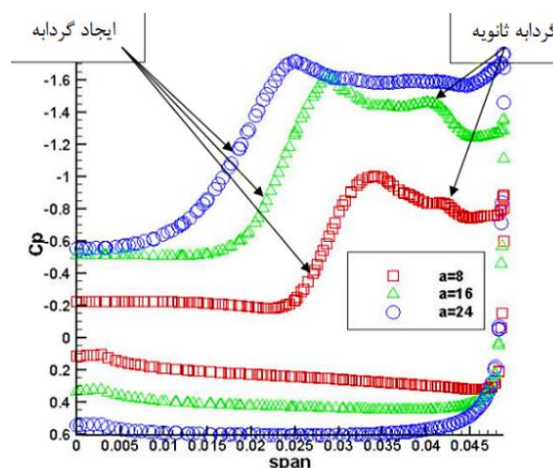
شکل ۷- مقایسه نمودارهای ضریب فشار بر حسب زاویه حمله در مقطع ۹۰٪، M=0.8 ، ۶۵
