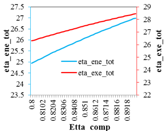
شکل ۴: تاثیر بازده کمپرسور بر بازده انرژی و بازده انرژی.
