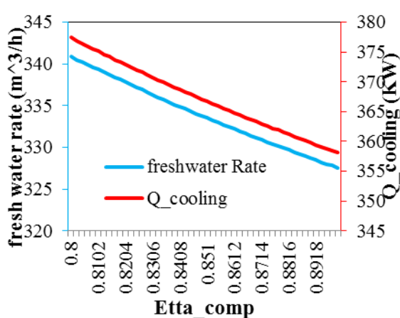
شکل ۷: تاثیر بازده کمپرسور بر دبی آب شیرین و سرمایه‌ش تولیدی سیستم.
