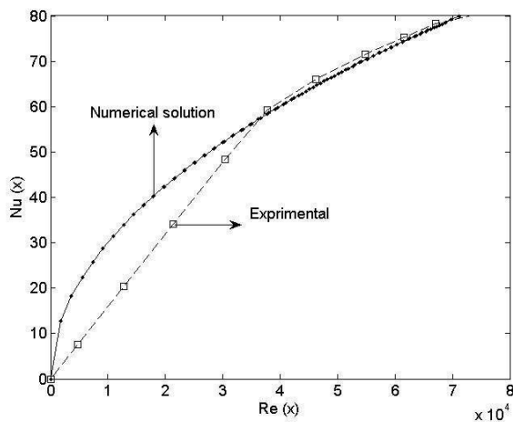
شکل ۹- نمودار تغییرات Nu(x) به Re(x) مقایسه‌ی Numerical solution به Experimental با Pr=0.71 و Re=1.72 \times 10^5 و Nu=122.54
