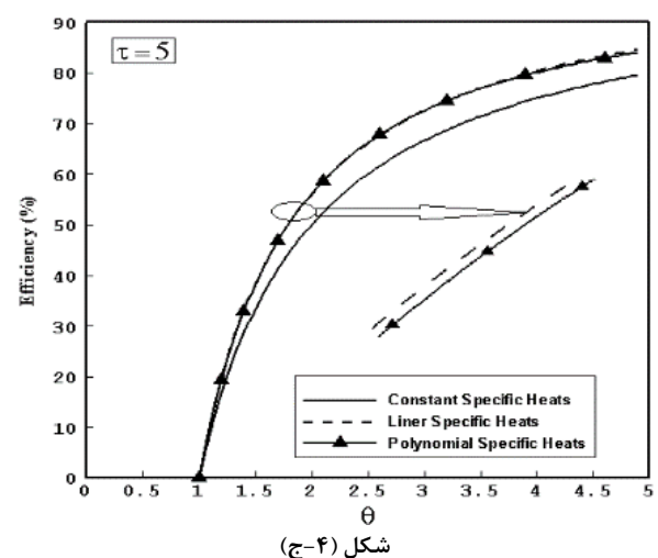
شکل ۴- منحنی تغییرات راندمان حرارتی سیکل برحسب \theta
