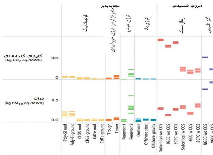
شکل ۳: گستره نتایج اثر تغییرات آب‌وهوایی و اثر ذرات برای فناوری‌ها و منابع انرژی مختلف [6]. جذب و ذخیره کربن دی‌اکسید CCS، کلسیم تلرید، مس ایندیم گالیوم سیلناید، چرخه ترکیبی گازی نیروگاه زغال‌سنگی، نیروگاه چرخه گاز طبیعی، نیروگاه بادی با فونداسیون ثقیل، نیروگاه بادی با فونداسیون فولادی، مخازن انرژی آبی به‌عنوان تخمین بالاتر، نیروگاه زغال‌سنگ پودری
