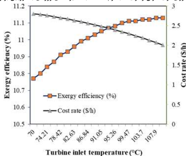
شکل ۷: بررسی تاثیر تغییرات دمای ورودی به توربین ( T_6 ) بر روی خروجی‌های سیستم
