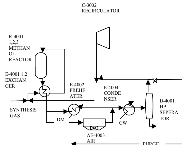
شکل ۱- شمای کلی واحد سنتز متانول پتروشیمی فن آوران
