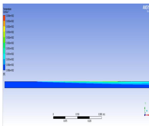
شکل ۶- الف. کانتور دما، ب. کانتور فشار، در داخل کانال برای شدت تابش خورشیدی ۱۱۰۰ وات بر متر مربع و رینولدز ۳۰۰۰
