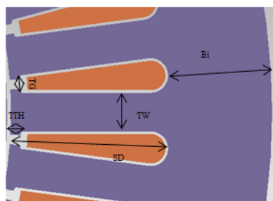
شکل ۱: ابعاد اساسی استاتور
