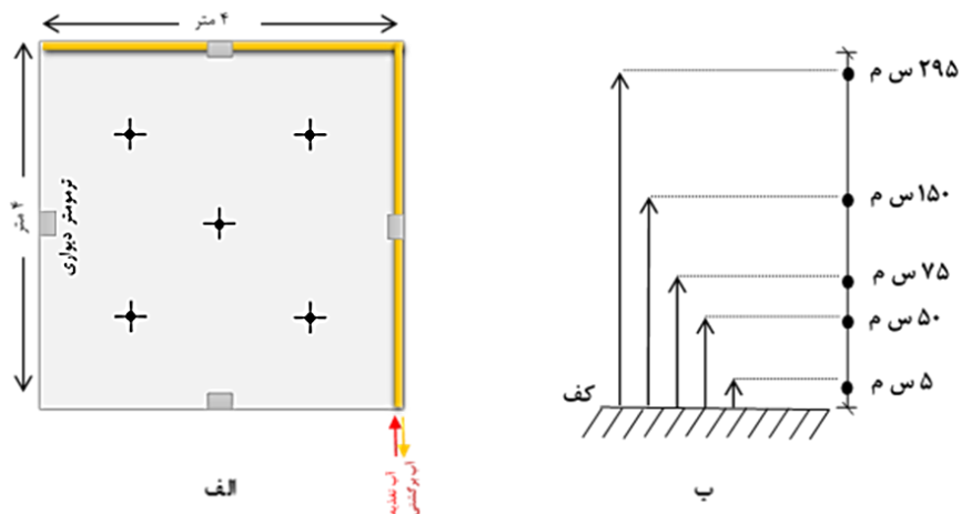
شکل ۴- (الف) پلان و مختصات چینش ترمومترهای داخل اتاق آزمون، (ب) ارتفاع ترمومترها از کف اتاق آزمون
