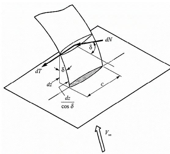
شکل ۱۲: نیروهای وارد بر المان پره [۲۹]
