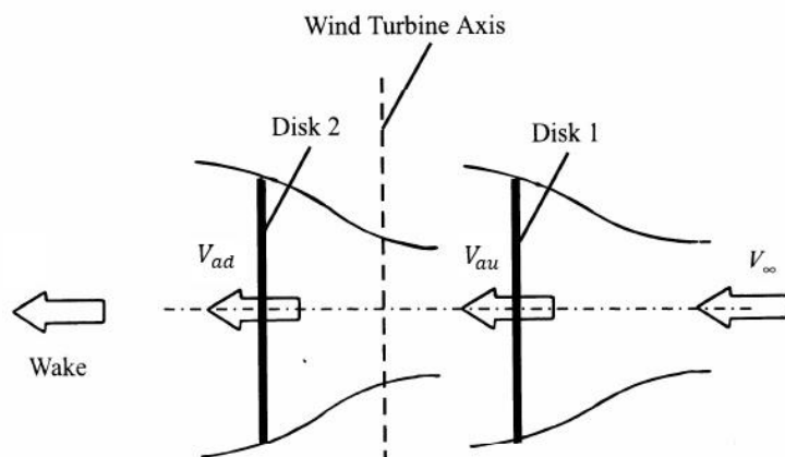
شکل ۷: مدل مومنتوم دو صفحه‌ای [۲۹]
