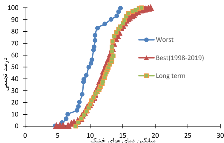
شکل ۳: نمونه ای از استفاده از روش ساندیا بدست آمده برای دمای هوای خشک طی سالهای ۱۹۹۸-۲۰۱۹ برای شهر تهران
