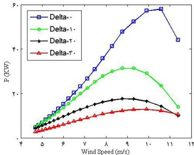
شکل ۹- تاثیر زاویه مخروطی بر منحنی توان توربین
