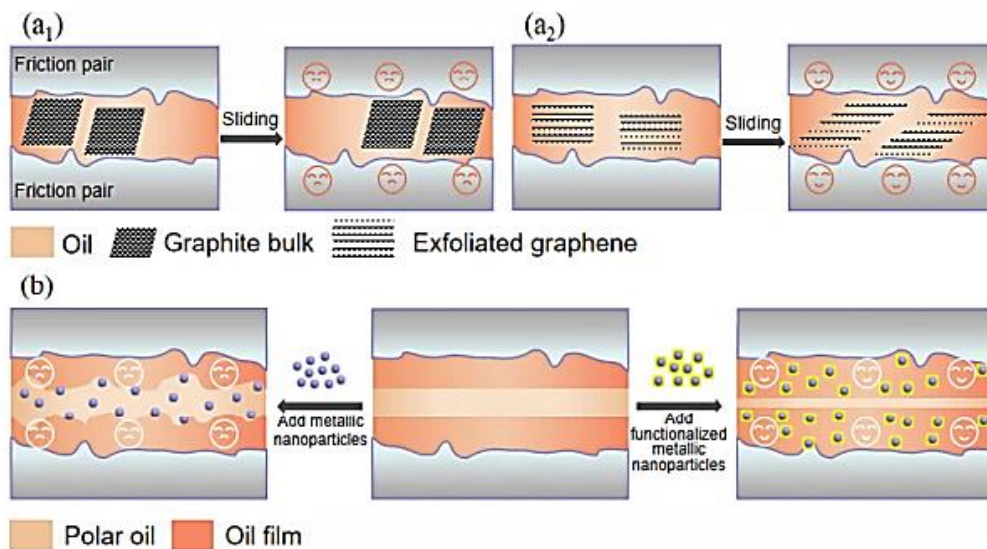
شکل ۴: نمودار مکانیسم‌ها
