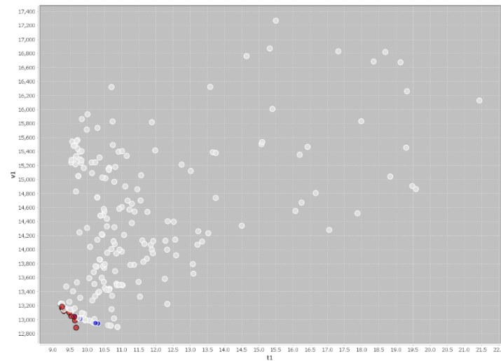
شکل ۶. نمودارهای پرتو بهینه‌سازی دو هدفه ساختمان در شهر تهران. در این شکل محور t1 نشان دهنده مقدار آسایش حرارتی ( PPD\% ) و محور t2 نشان دهنده انرژی کل ( kWh ) می باشند.
