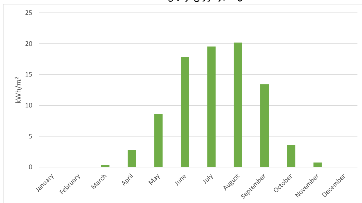
شکل ۵- بار حرارتی سرمایش فضا \text{kWh/m}^2
