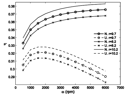
شکل ۱۲) نمودار راندمان-سرعت زاویه‌ای لنگ، در مکانیزمهای مرسوم و پیشنهادی و به ازای تغییرات نسبت تراکم
