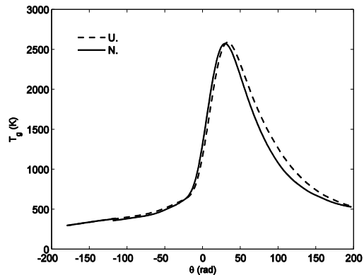
شکل ۶) نمودار تغییرات دمای گازهای درون سیلندر (با استفاده از نتایج بخش ۴) در مکانیزمهای مرسوم و پیشنهادی
