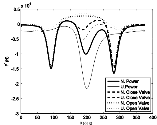
شکل ۱۶) نمودار نیروهای وارده بر شاتون-زاویه لنگ، در شرایط با احتراق و بدون احتراق با سوپاپ بسته و باز در مکانیزمهای مرسوم و پیشنهادی و به ازای \omega = \dot{\theta} = 3500 \text{ rpm} و l = 1.05R
