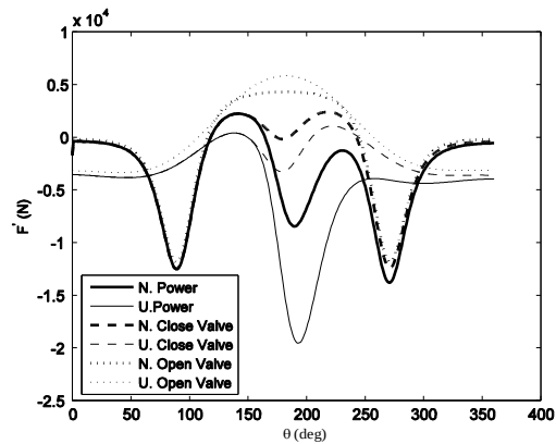
شکل ۱۵) نمودار نیروهای وارده بر شاتون-زاویه لنگ، در شرایط با احتراق و بدون احتراق با سوپاپ بسته و باز در مکانیزمهای مرسوم و پیشنهادی و به ازای \omega = \dot{\theta} = 4500 \text{ rpm}
