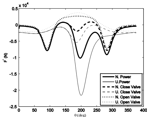
شکل ۱۴) نمودار نیروهای وارده بر شاتون-زاویه لنگ، در شرایط با احتراق و بدون احتراق با سوپاپ بسته و باز در مکانیزمهای مرسوم و پیشنهادی و به ازای \omega = \dot{\theta} = 3500 \text{ rpm}
