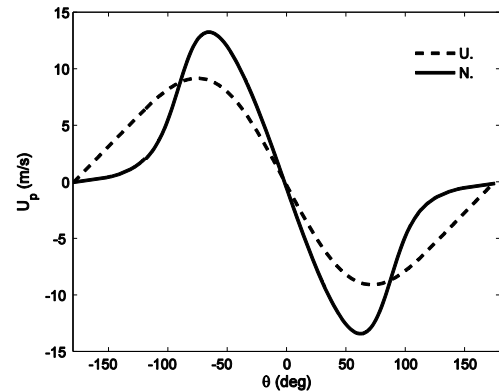
شکل ۵) نمودار تغییرات سرعت پیستون در بازه ۳۶۰ درجه چرخش میل لنگ در مکانیزمهای مرسوم و پیشنهادی
