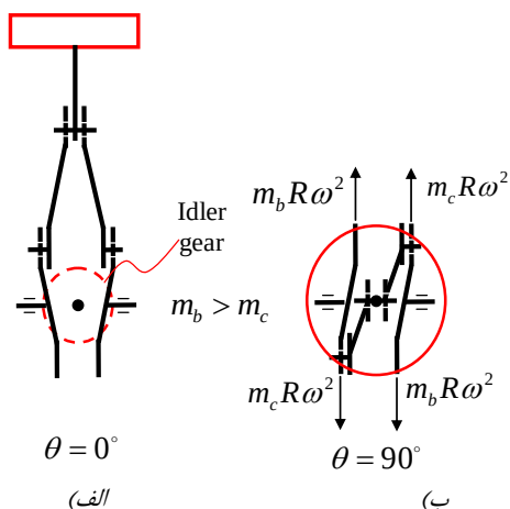
شکل (۲) نحوه توازن کامل گشتاورها در مکانیزم پیشنهادی در نمایه‌های (الف) روبرو (ب) بالا
