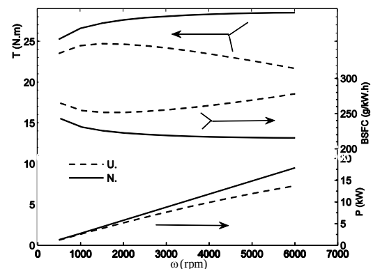
شکل ۱۳) نمودارهای تغییرات گشتاور ترمزی، مصرف ویژه سوخت ترمزی و توان خروجی ترکیبهای پیشنهادی و مرسوم
