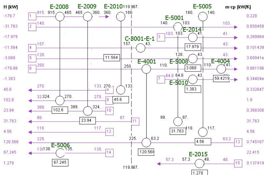
شکل ۲- دیاگرام شبکه منتخب واحد متانول نمونه در وضعیت موجود (ماخذ: اطلاعات اخذ شده از واحد و محاسبات محققین)
