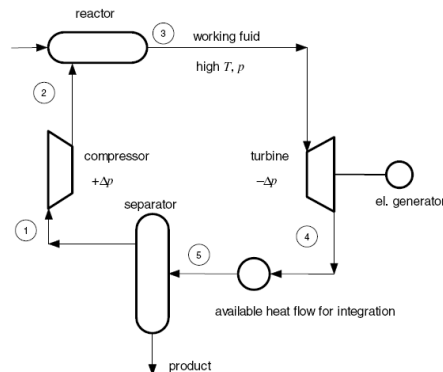
شکل ۳- نحوه یکپارچه سازی توربین گاز با راکتور شیمیایی [۵۰]
