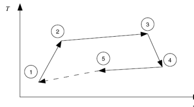
شکل ۴- نمودار ساده شده T-S در سیکل توربین گاز نشان داده شده در شکل (۳) [۵۰]
